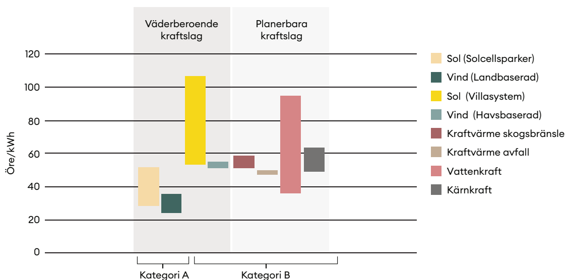
LCOE-intervall för olika tekniker.
